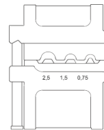
Die profile
