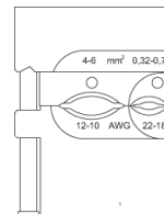
Die profile
