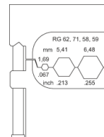
Die profile
